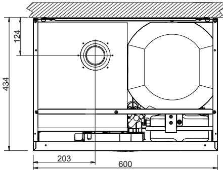
εικ. 45- Κάτωψη
