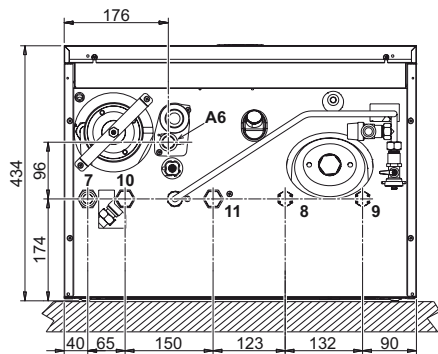
εικ. 46- Άνοψη
