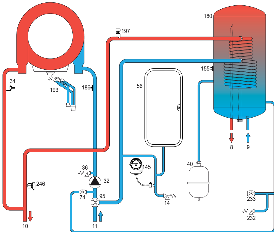
fig. 48- Circuito hidráulico
