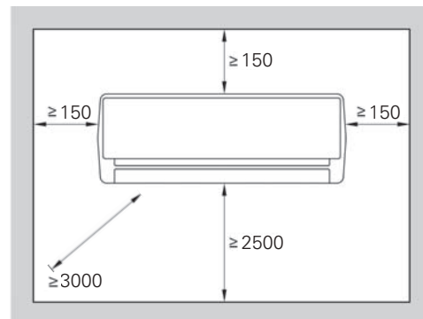
Čelní pohled
